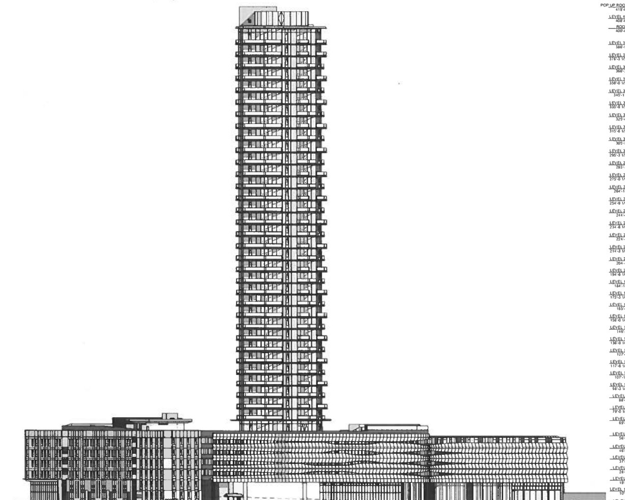
MAKAI ELEVATION
